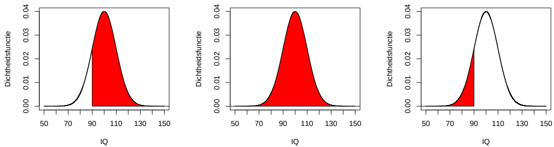
Figuur 5.12: Illustratie van formule (5.9) met x = 90 . De gekleurde oppervlakte van de figuur links geeft de kans P(IQ > 90) weer. De gekleurde oppervlakte van de figuur in het midden is gelijk aan 1, zie formule (5.8). De gekleurde oppervlakte voor de figuur rechts geeft de kans P(IQ \leq 90) weer. Het verschil in oppervlakte tussen de figuur in het midden en de figuur rechts is gelijk aan de oppervlakte van de figuur links.
