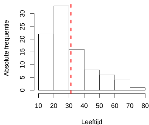
Figuur 3.1: Een histogram van de variabele Leeftijd met aanduiding van het gemiddelde.
