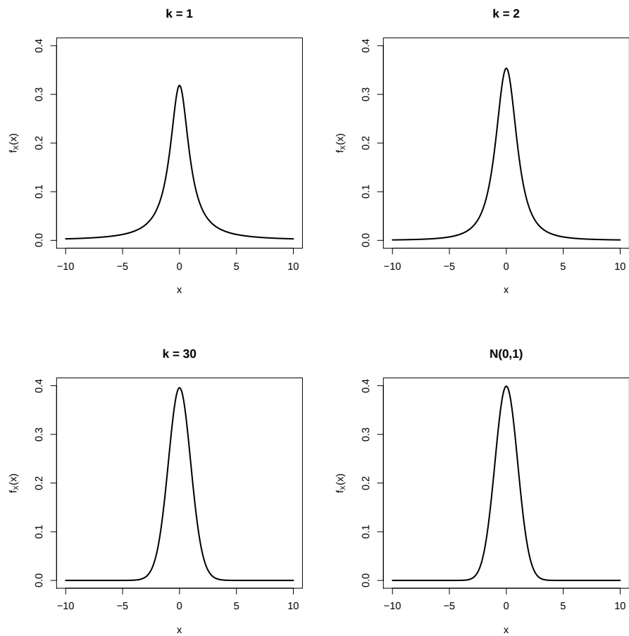
Figuur 5.22: De dichtheidsfunctie van een t-verdeling met k vrijheidsgraden voor verschillende waarden van k . Naarmate k toeneemt, zal de dichtheidsfunctie meer gelijken op die van een standaard normale (figuur rechtsonder).
