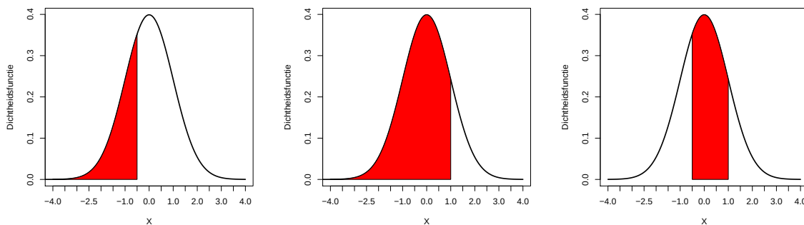
Figuur 5.17: De grafische weergave van de kansen P(X \leq -0.5) (gekleurde oppervlakte figuur links), P(X \leq 1) (gekleurde oppervlakte figuur midden) en P(-0.5 \leq X \leq 1) (gekleurde oppervlakte figuur rechts). Merk op dat de gekleurde oppervlakte in de figuur rechts gelijk is aan het verschil in gekleurde oppervlakte van de figuur in het midden en de figuur links. Dit komt overeen met de eigenschap dat P(-0.5 \leq X \leq 1) = P(X \leq 1) - P(X \leq -0.5) .
