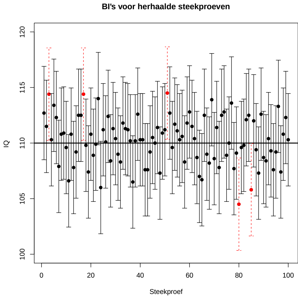
Figuur 7.5: Visualisatie van de 95% betrouwbaarheidsintervallen voor de 100 verschillende steekproeven met n = 50 . De horizontale volle lijn duidt het populatiegemiddelde \mu = 110 aan en de stippen duiden de steekproefgemiddelden aan. De rode intervallen in stippellijn snijden de horizontale lijn niet en bevatten bijgevolg het populatiegemiddelde niet. Er zijn 95 van de 100 intervallen zwart gekleurd, wat overeenkomt met 95%.
