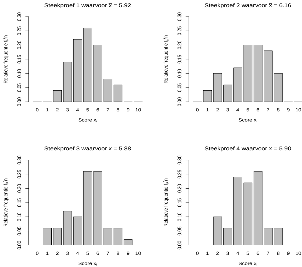
Figuur 6.3: Staafdiagram van de score op de Benton Visual Retention Test en de gemiddelde score voor 4 verschillende steekproeven met n = 50 .
