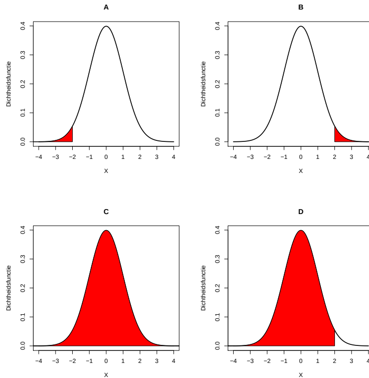
Figuur 5.19: Figuur A: grafische weergave van de kans P(X \leq -2) . Figuur B: grafische weergave van de kans P(X > 2) (uit Figuur 5.18 weten we dat deze kans gelijk is aan P(X \leq -2) ). Figuur C: de volledige oppervlakte is altijd gelijk aan 1. Figuur D: grafische weergave van de kans P(X \leq 2) . Merk op dat de gekleurde oppervlakte in figuur B gelijk is aan het verschil in gekleurde oppervlakte van figuur C en D (dus P(X > 2) = 1 - P(X \leq 2) ) en dat de gekleurde oppervlakte van figuur B gelijk is aan de gekleurde oppervlakte van figuur A (dit is P(X > 2) = P(X \leq -2) ). Dit kunnen we samenbrengen tot de eigenschap P(X \leq -2) = 1 - P(X \leq 2) .
