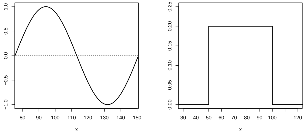
Figuur 5.11: Links: functie die geen dichtheidsfunctie kan zijn omdat ze negatieve waarden aanneemt. Rechts: functie die geen dichtheidsfunctie kan zijn omdat de volledige oppervlakte onder de dichtheidsfunctie verschillend is van 1.
