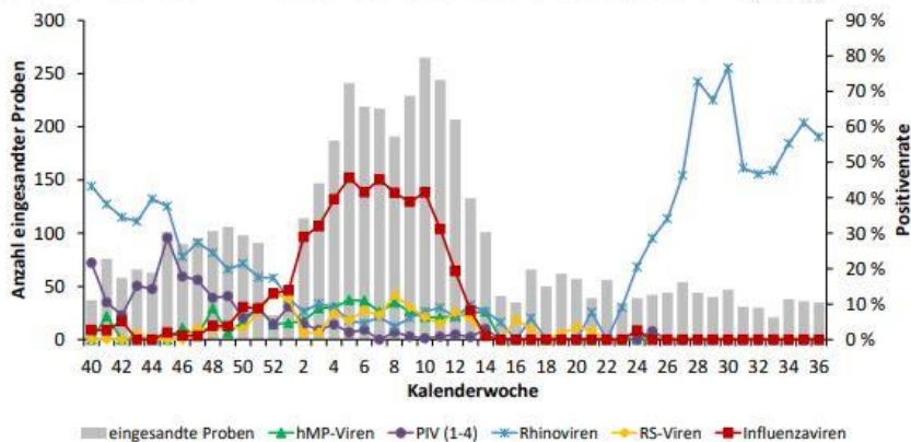
Abb. 3: Anteil positiver Influenza-, RS-, hMP-, PI- und Rhinoviren an allen im Rahmen des Sentinels eingesandten Proben (Positivrate, rechte y-Achse, Linien) sowie die Anzahl der an das NRZ für Influenzaviren eingesandten Sentinelproben (linke y-Achse, graue Balken) von der 40. KW 2019 bis zur 36. KW 2020.
